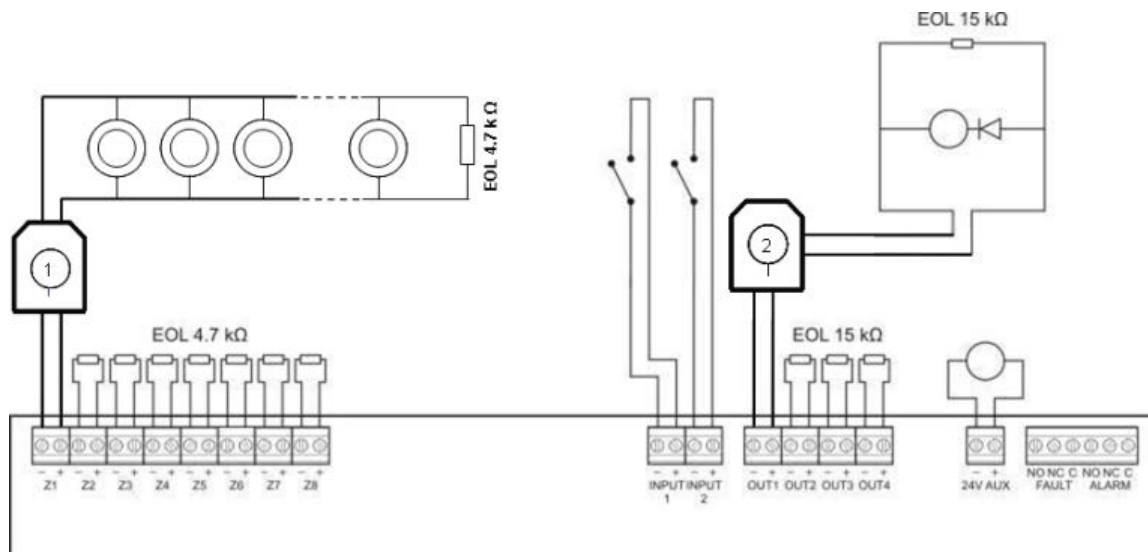
Rysunek 7: Iskrobezpieczne złącze systemu przeciwpożarowego
