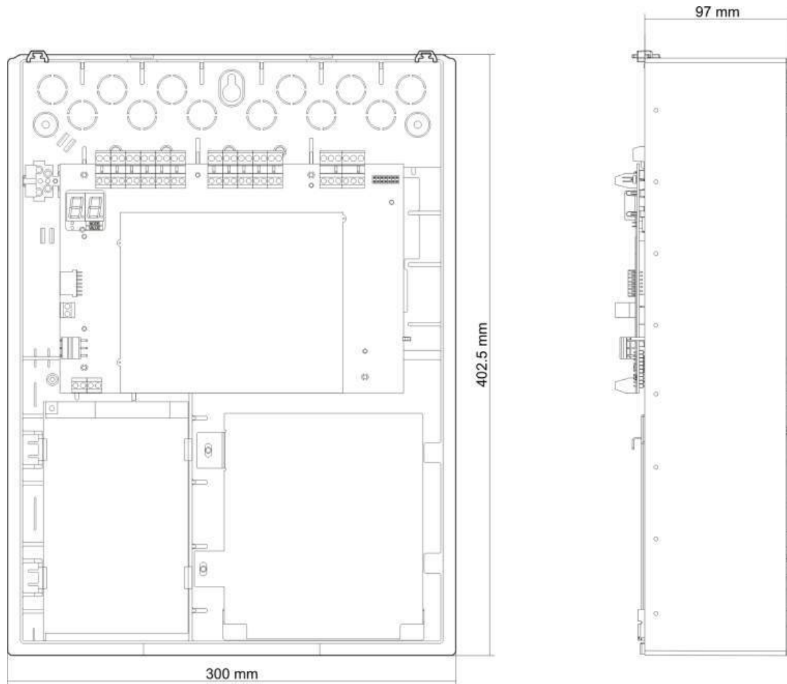
Rysunek 22: Centrale dwu- i czteroliniowe bez pokrywy
