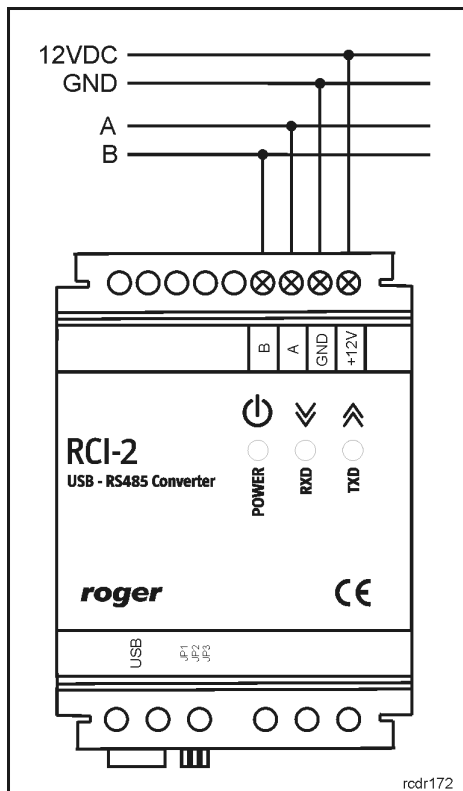
Rys. 1 Podłączenie RCI-2 do systemu RACS
