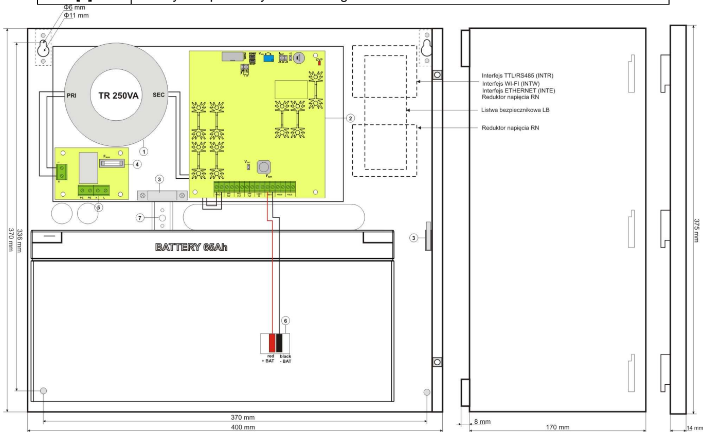
Rys.3. Widok zasilacza.
