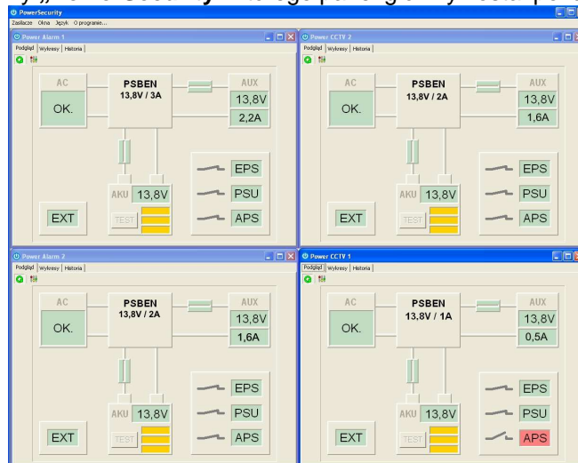
Rys. 16. Panel główny programu „Power security”.
