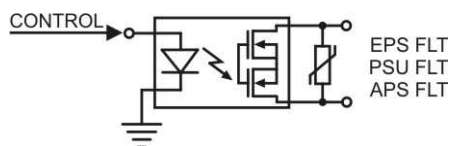
Rys. 6. Schemat elektryczny wyjść technicznych.
